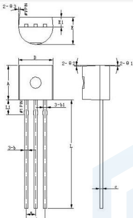
TO-92-A1
