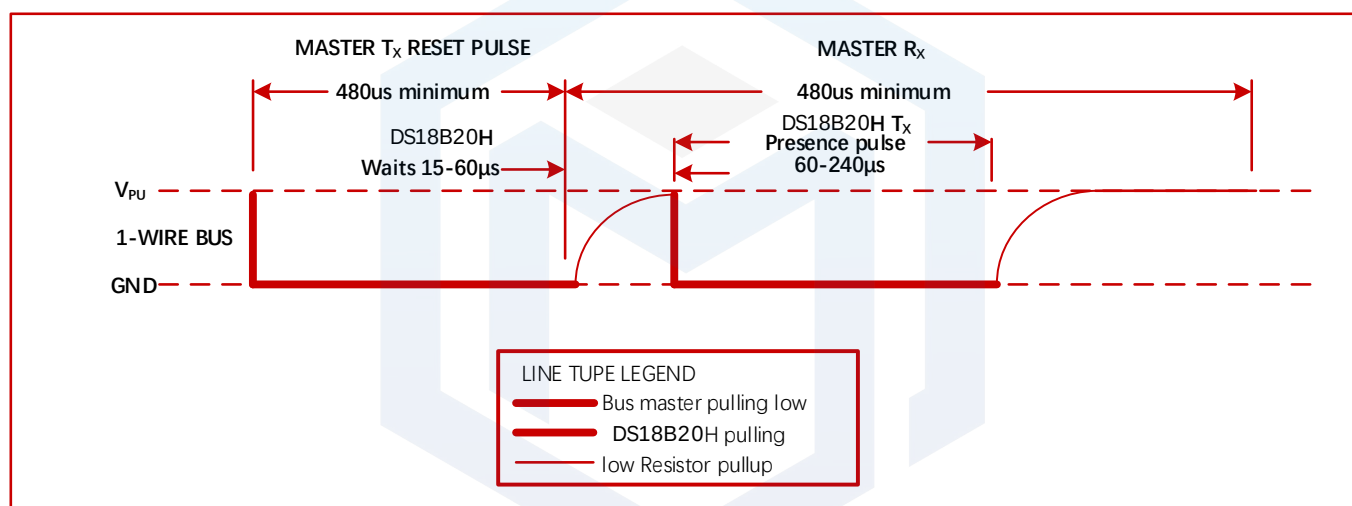
图 13. 初始化序列
