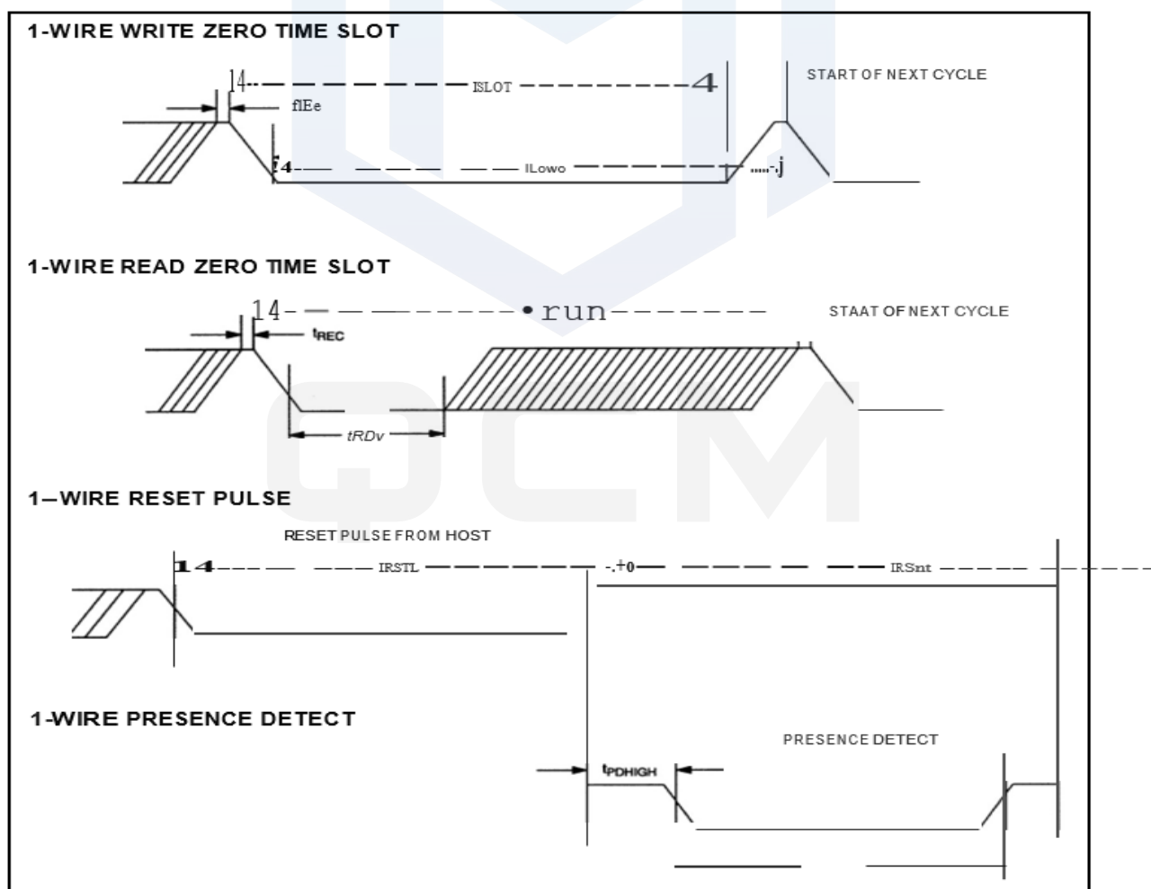
图 18. 时序
