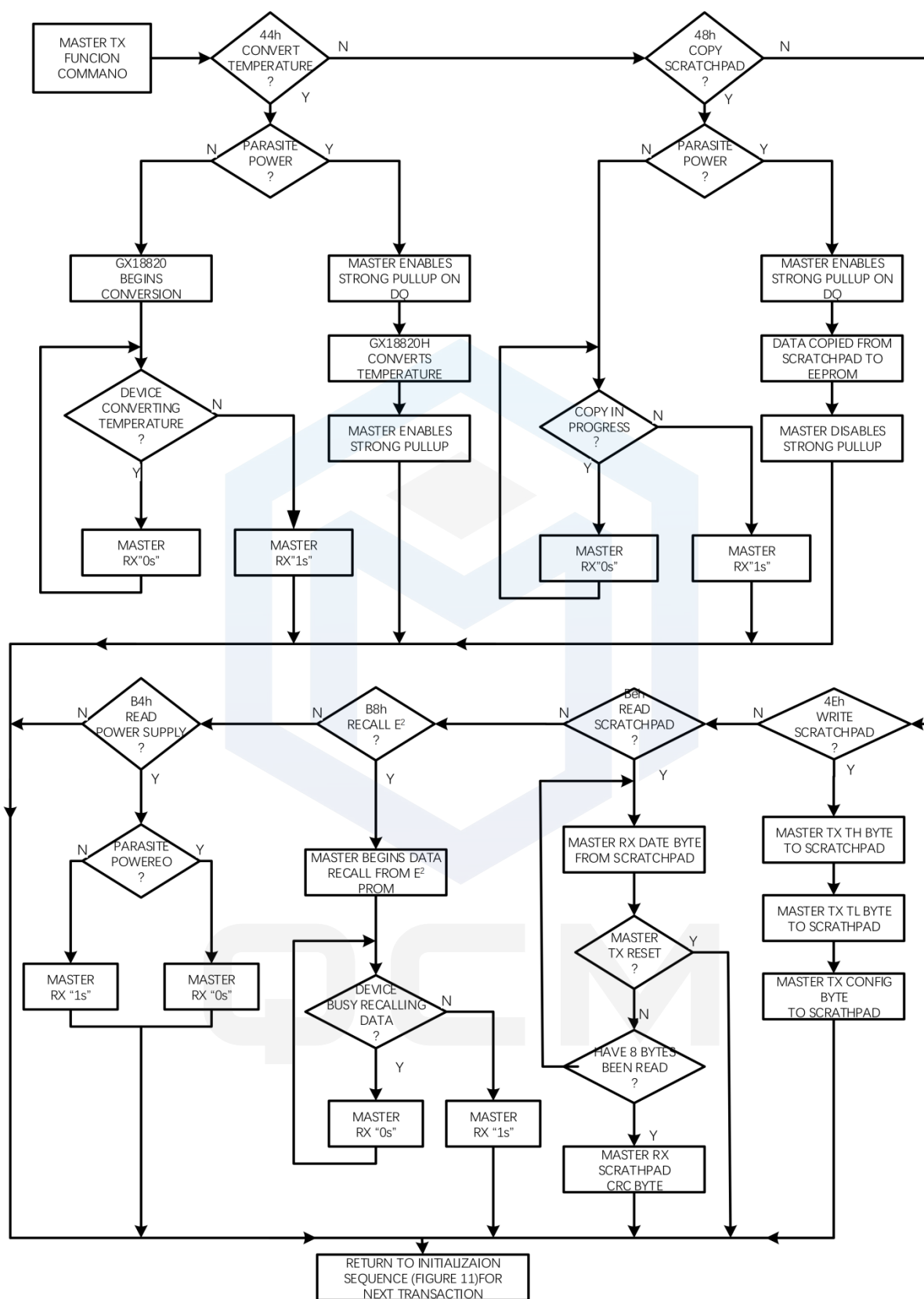
图 12. DS18B20功能指令流程图
